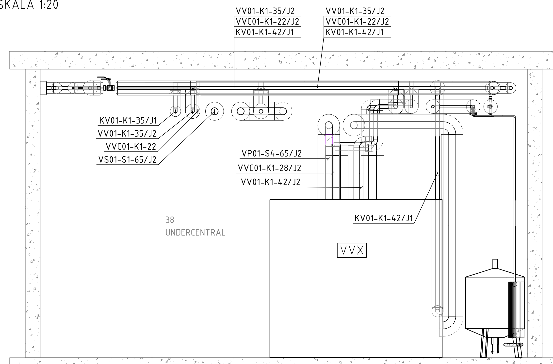
SEKTION 1 SKALA 1:20
